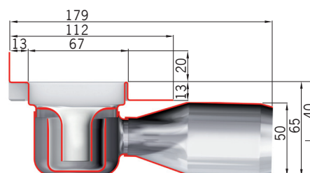
Plitka ugradnja sa vertikalnom prirubnicom
