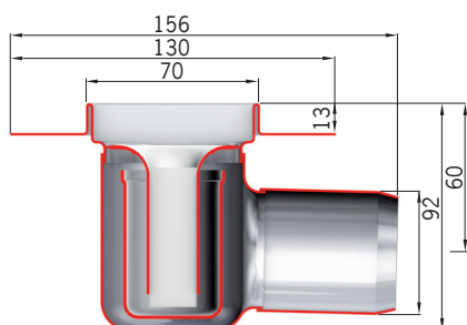
Normalna ugradnja sa plitkim hidroizolacijskim premazom
