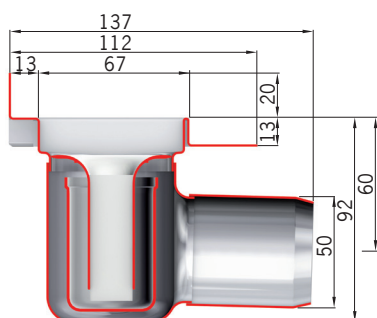
Normalna ugradnja sa vertikalnom prirubnicom
